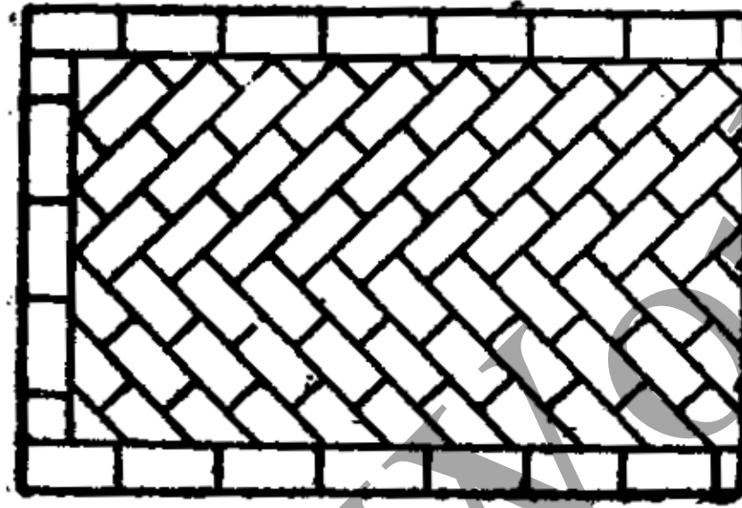
Fig 11.24 Zigzag Bond
