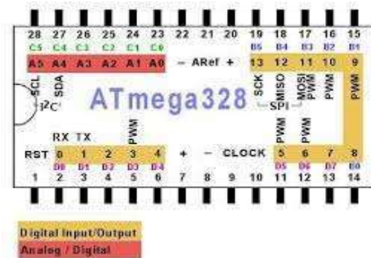
Fig:8 ATMEGA328
